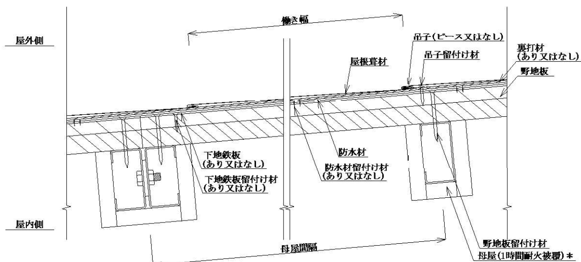
[B - B' 断面詳細図]
